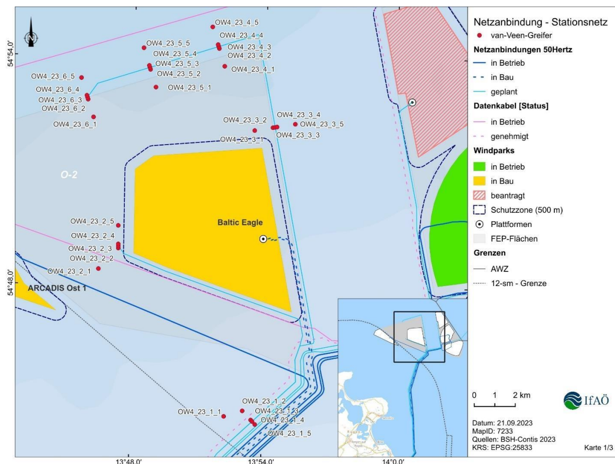
Abbildung 2: Verlauf des geplanten Netzanbindungssystems OST-2-4 durch die deutsche AWZ mit dem Stationsnetz der Untersuchungen mittels van-Veen-Greifer im Herbst 2023 (Quelle: Unterlage M)
